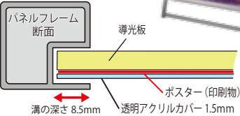
一断面図一
